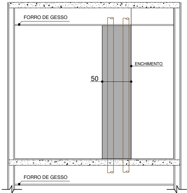
VISTA 1
