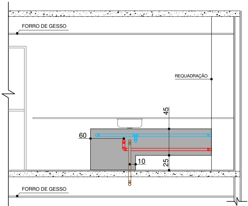
VISTA 1
