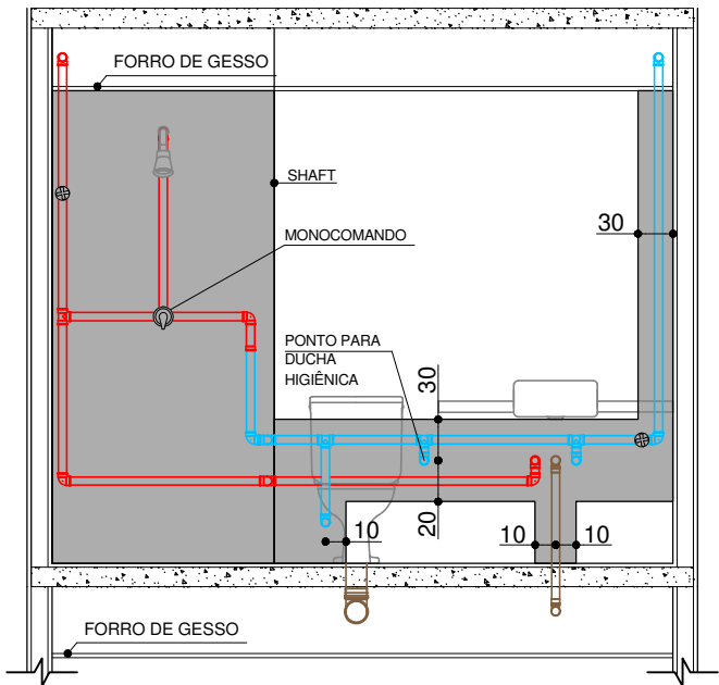
VISTA 1
