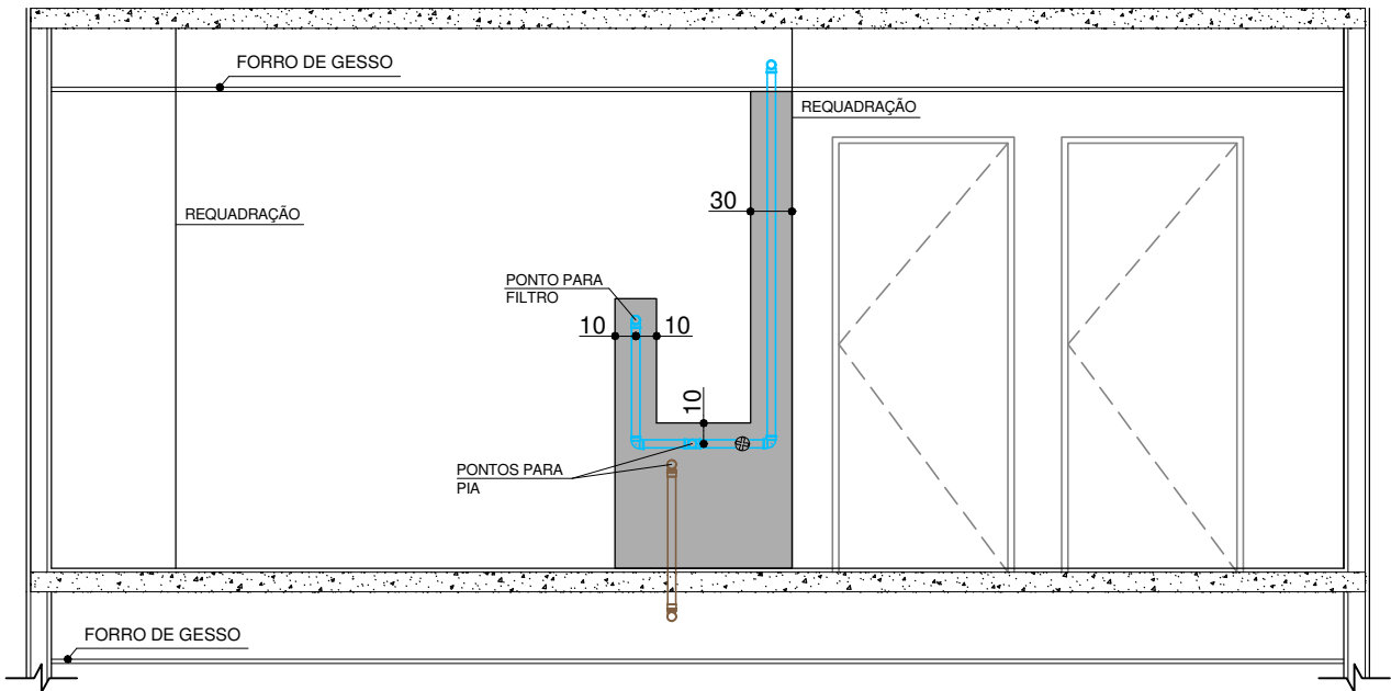
VISTA 1
