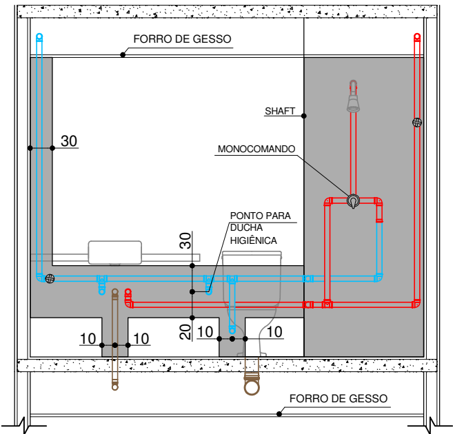
VISTA 1
