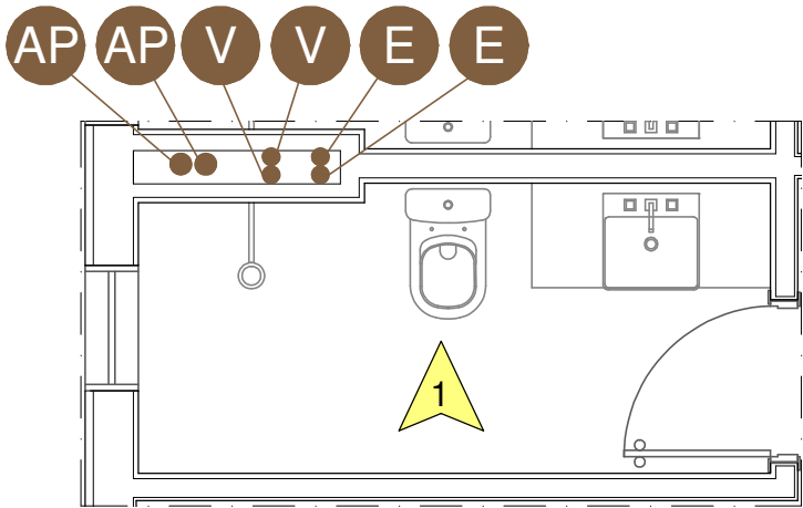
PLANTA
