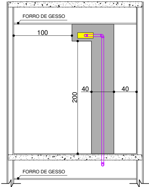
VISTA B
