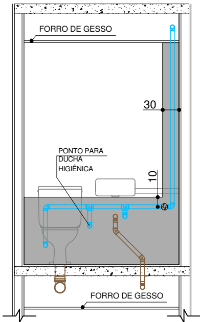
VISTA 1
